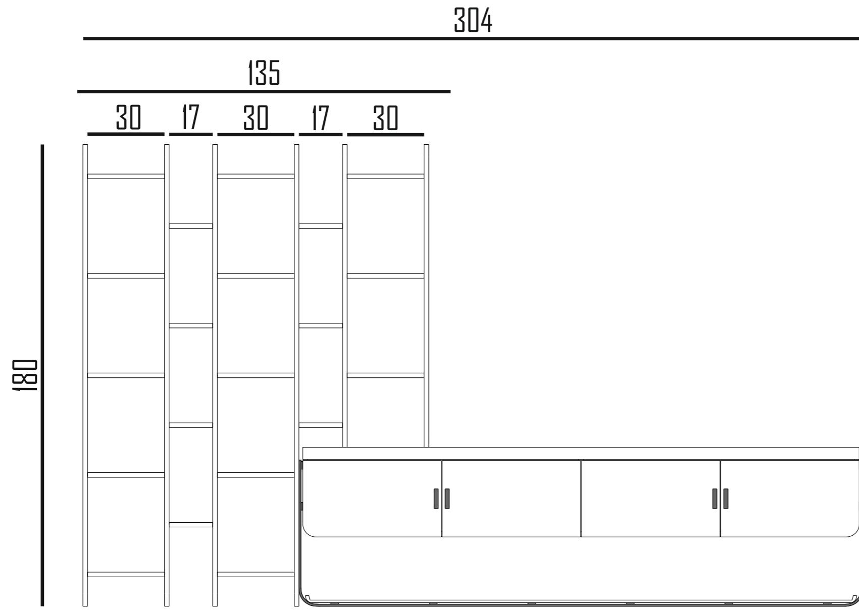
ÖN GÖRÜNÜS FRONT VIEW
