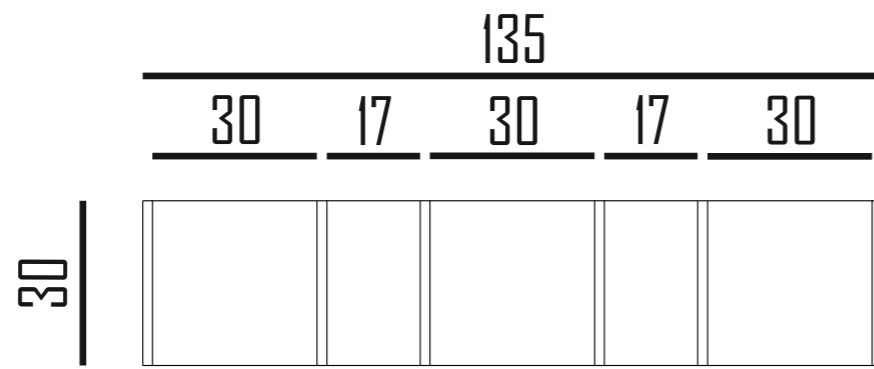
ÜST GÖRÜNÜS TOP VIEW
