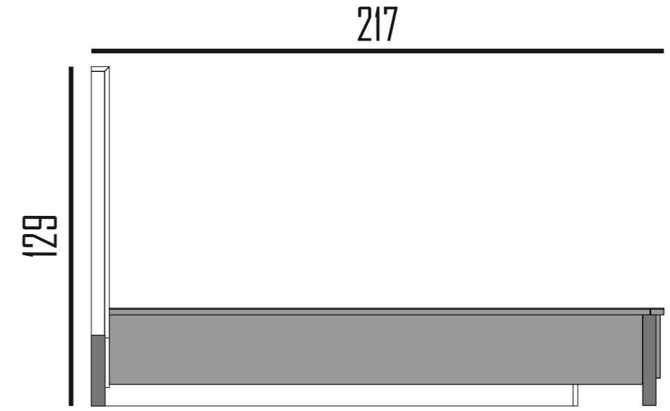
YAN GÖRÜNÜS SIDE VIEW
