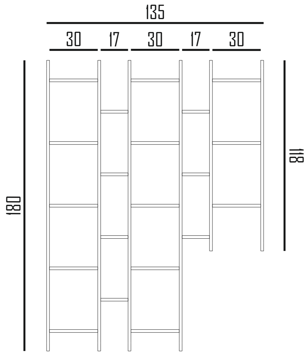
ÖN GÖRÜNÜS FRONT VIEW
