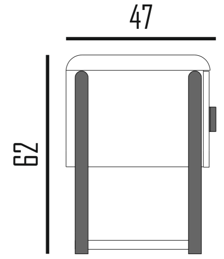
YAN GÖRÜNÜS SIDE VIEW
