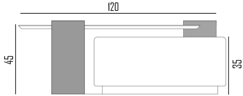
ÖN GÖRÜNÜS FRONT VIEW
