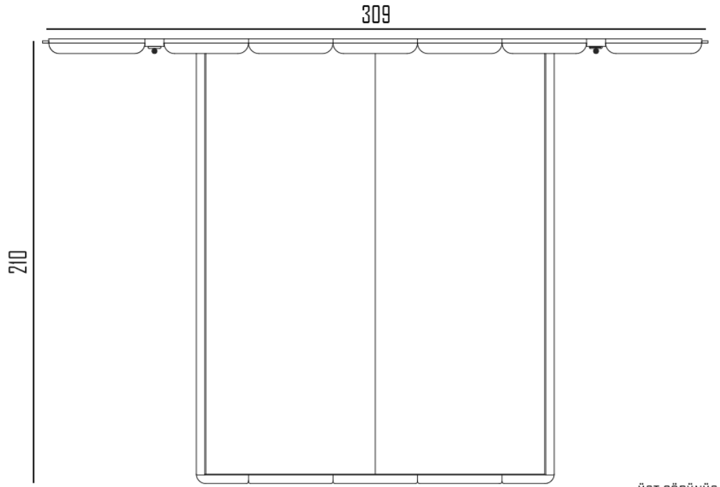
ÜST GÖRÜNÜS TOP VIEW
